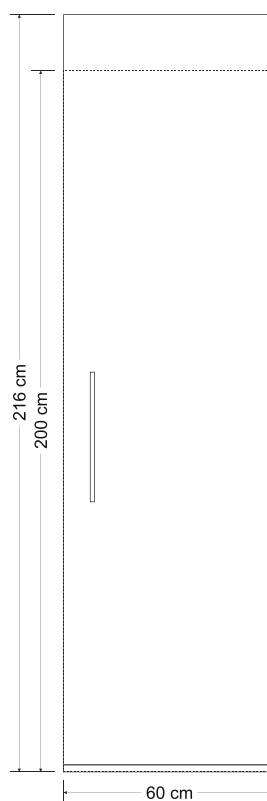
esquisse: HO - H2000/H2160
